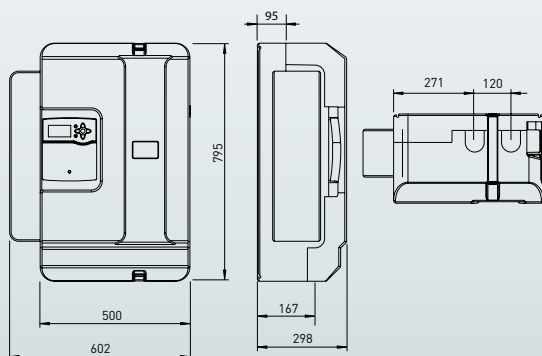
SCHEMA INSTALLATIVO INSTALLAZIONE SINGOLA
