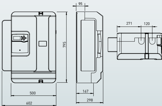
SCHEMA INSTALLATIVO INSTALLAZIONE SINGOLA
