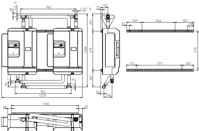
SCHEMA DIMENSIONALE INSTALLAZIONE IN CASCATA
