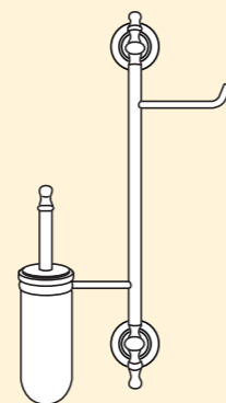
L/135 cm 31x48hx10p Colonna attrezzata WC c/ p. rotolo e p. scopino Fitted column for WC w/toilet paper holder and brush holder Eingerichteter Hochschrank WC mit Papierrollenhalter und WC- Bürstenhalter Colonne WC équipée avec porte-rouleau et balayette оборудованная стойка для унитаза с держателями туалетной бумаги и ёршика.
