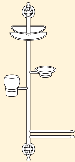
L/133 cm 33x90hx10p Colonna attrezzata lavabo c/ mensolina, p. sapone, p. bicchiere e 2 p. asciugamani Fitted column for wash basin w/small shelf, soap dish, glass holder and 2 towel rails Eingerichteter Hochschrank für Waschbecken mit kleiner Konsole, Seifenschale, Glashalter und 2 Handtuchhalter Colonne lavabo équipée avec tablette, porte-savon, porte-verre et 2 porte - serviettes стойка умывальника с полочкой, мыльницей, подстаканником и двумя вешалками для полотенец
