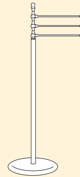
L/123 Ø base cm 26 - h cm 90 Piantana a 3 bracci orientabili Towel stand with 3 swivel arms Ständer mit 3 ausrichtbaren Armen Montant avec 3 bras pivotants Стойка с 3 поворотными рычагами
